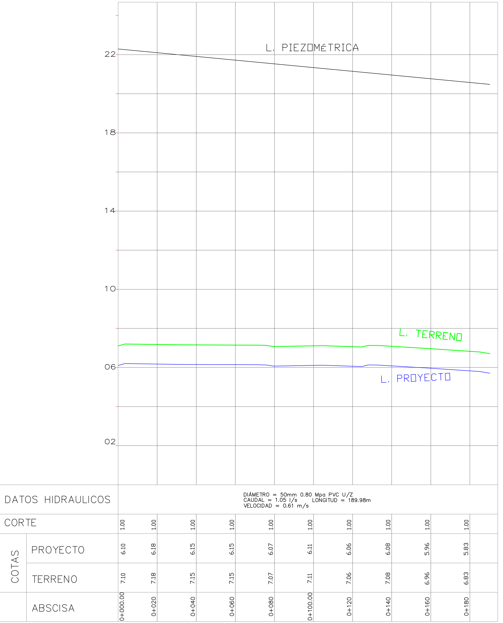
PERFIL LONGITUDINAL RAMAL "R42"
