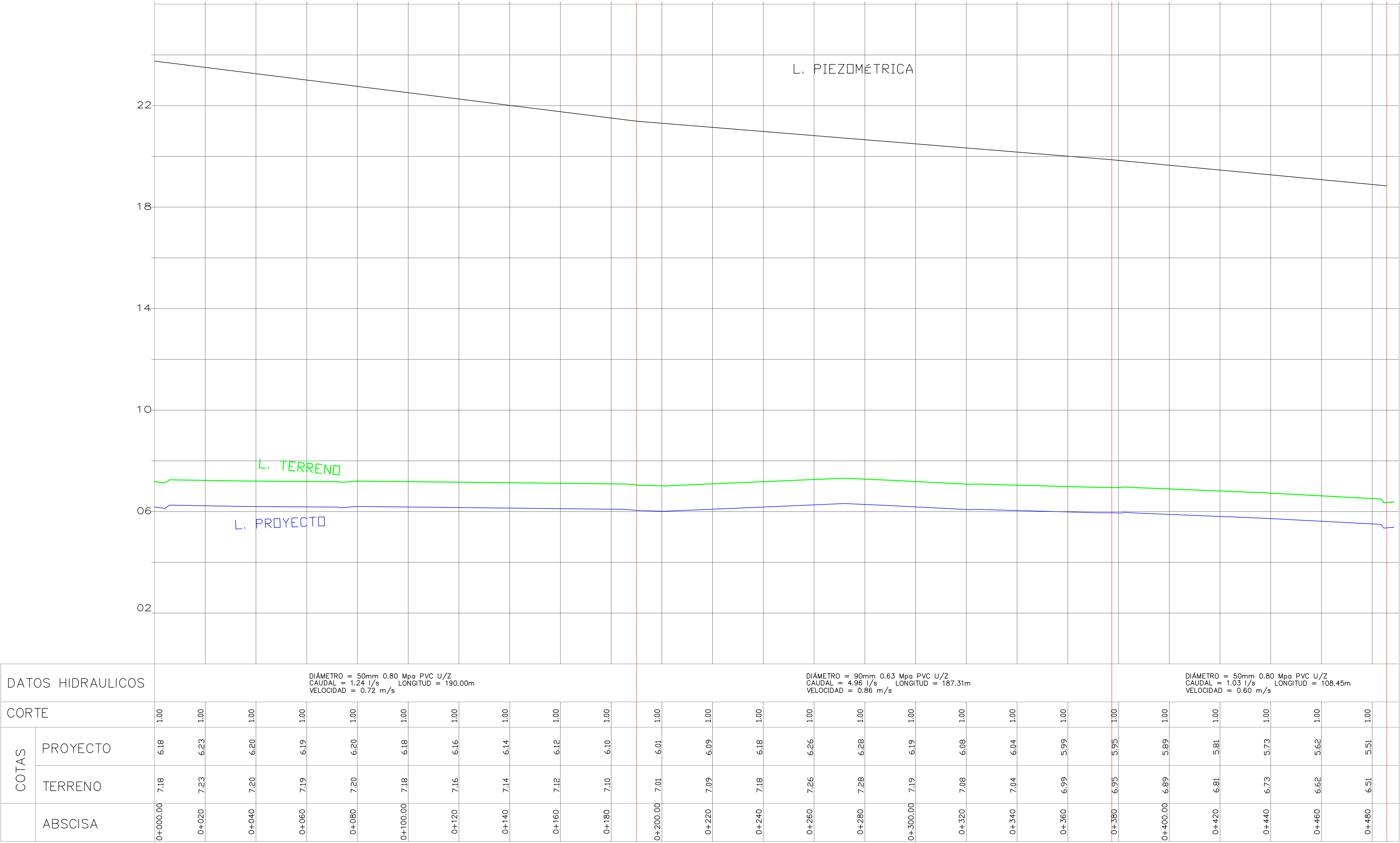
PERFIL LONGITUDINAL RAMAL "R41"
